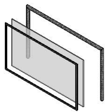
VITRAGE DE PORTE AVEC JOINTS D'ÉTANCHÉITÉ
